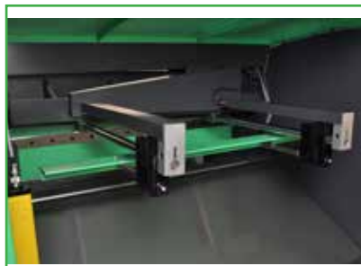
Hochpräziser, motorisierter Hinteranschlag mit einer Arbeitslänge bis zu 635 mm.
